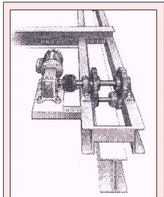
Las grúas Top Runner ruedan sobre la viga de la Vía Carrilera, eliminando el costoso riel ASCE. Son muy similares a las grúas descolgadas, que ruedan en el inferior de la viga de la vía carrilera
